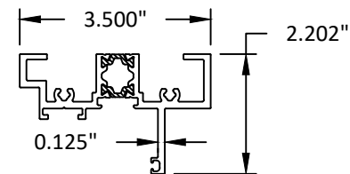
3 DOOR STILE/RAIL
