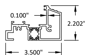
4 HD ASTRAGAL
